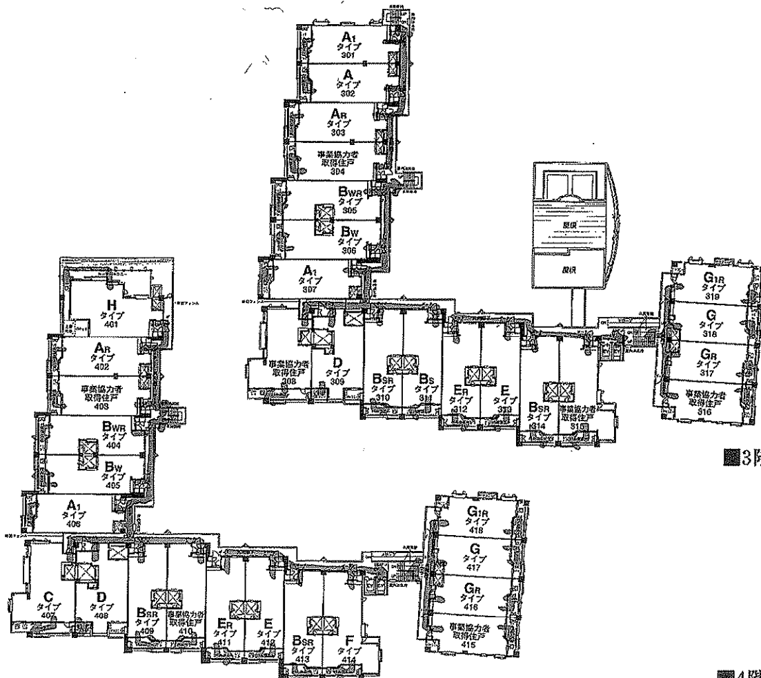
■4階平面図
